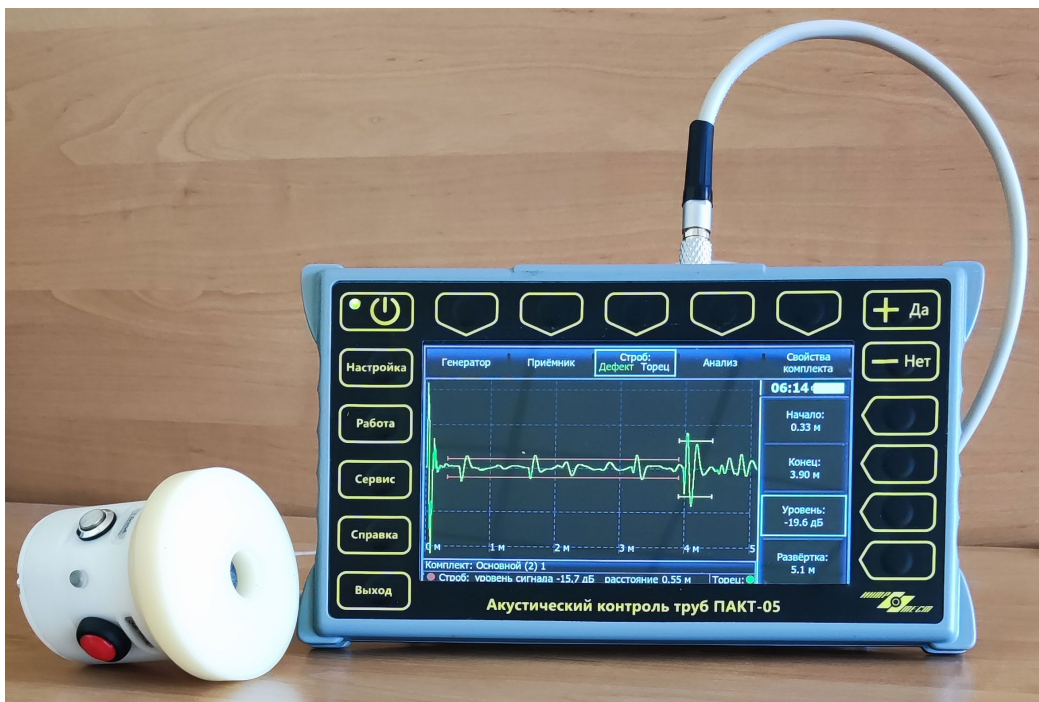
Прибор ПАКТ-05
